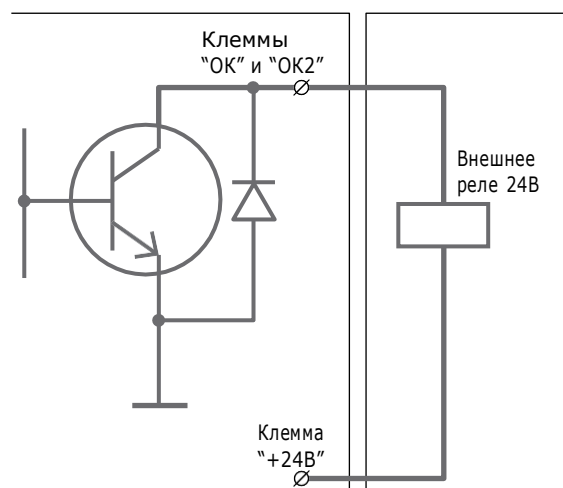
Рисунок 7. Подключение промежуточного реле
