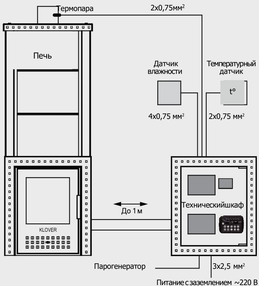
Схема подключения газового оборудования
