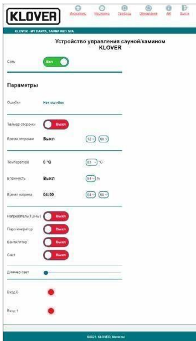
Рисунок 9. Web-интерфейс Устройства
