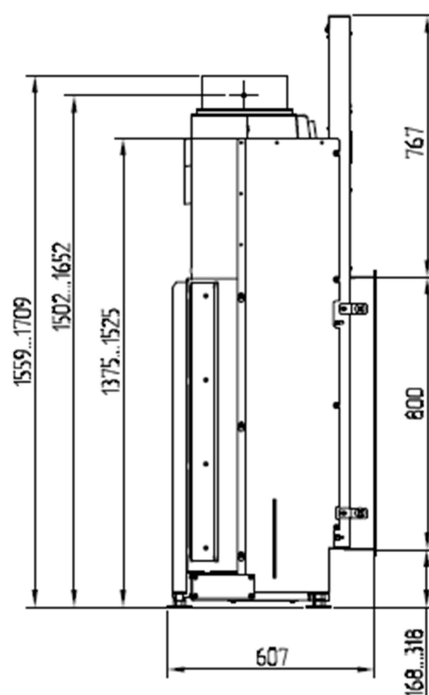
A-A
