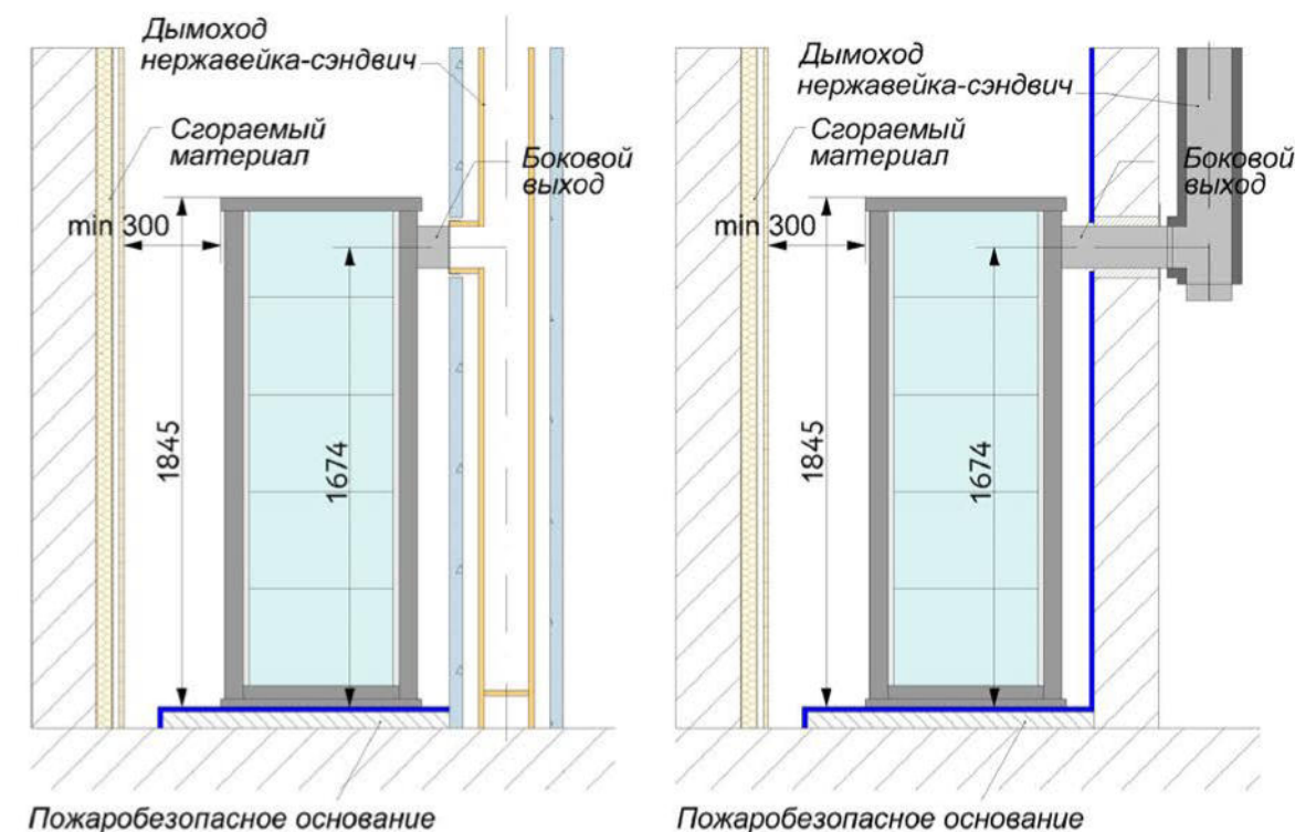
Схематичный чертеж подключения KLV-RT-50RV 310s к дымоходу
